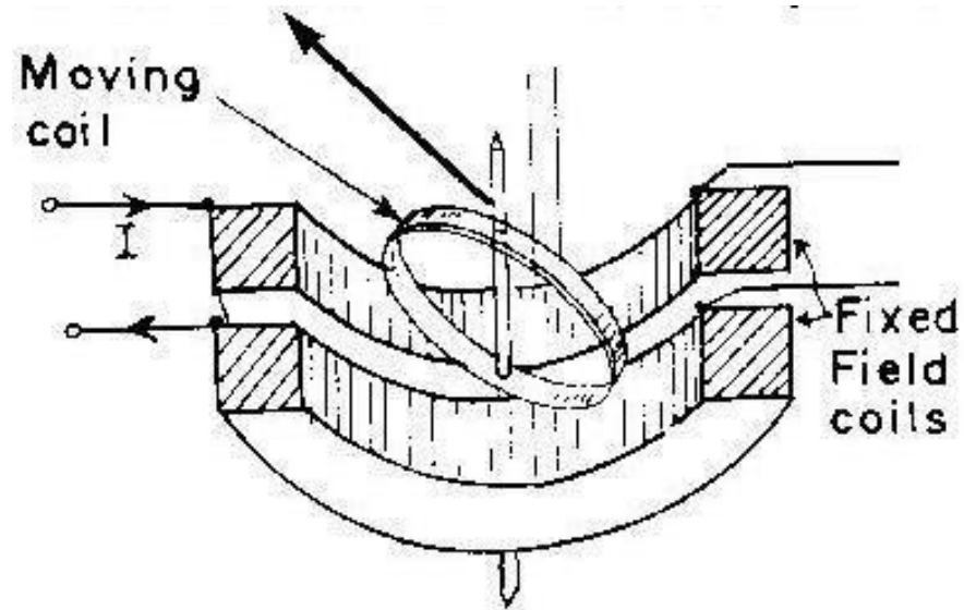
Fig. 11.2. Dynamometer wattmeter.
