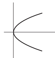
(b) Parabola
